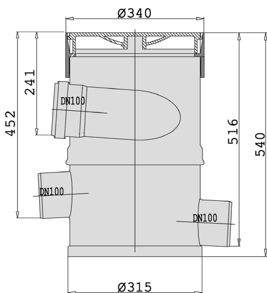
WF 20 02 - WFF 100 SANS REHAUSSE
